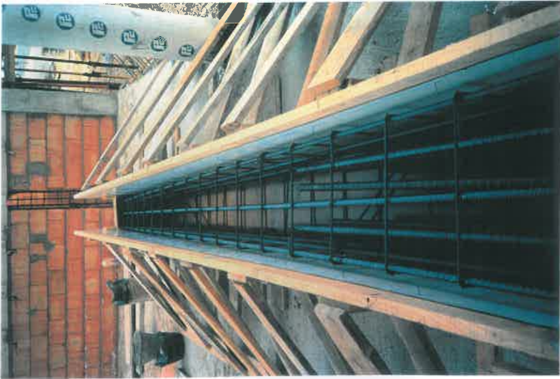
ENCOFRADO DEL MONOLITO
